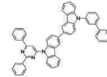
[化学式 A-9]
