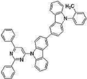
[化学式 B-20]
