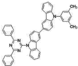
[化学式 B-9]
