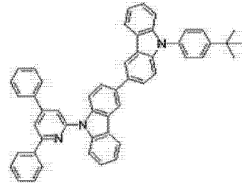
[化学式 B-16]
