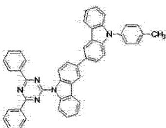
[化学式 B-4]
