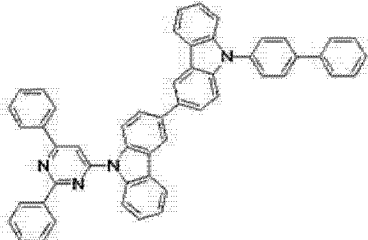
[化学式 A-7]
