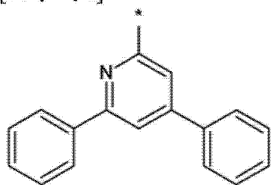
[化学式 6]
