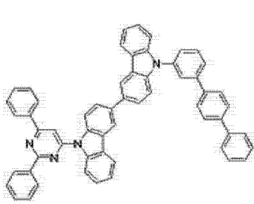
[化学式 A-25]
