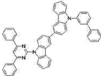
[化学式 A-11]
