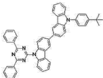
[化学式 B-14]
