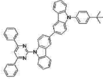
[化学式 B-15]
