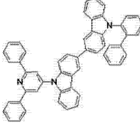
[化学式 A-33]
