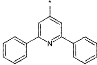
[化学式 5]
