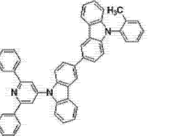
[化学式 B-21]
