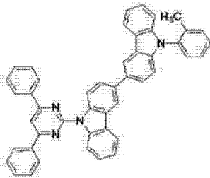
[化学式 B-18]
