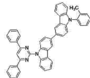
[化学式 B-18]
