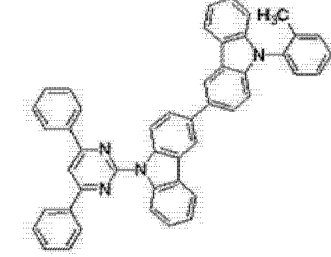
[化学式 B-18]
