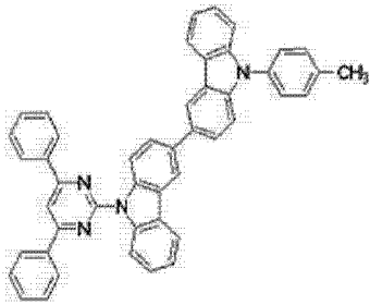
[化学式 B-5]
