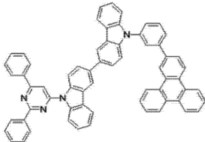
[化学式 A-36]
