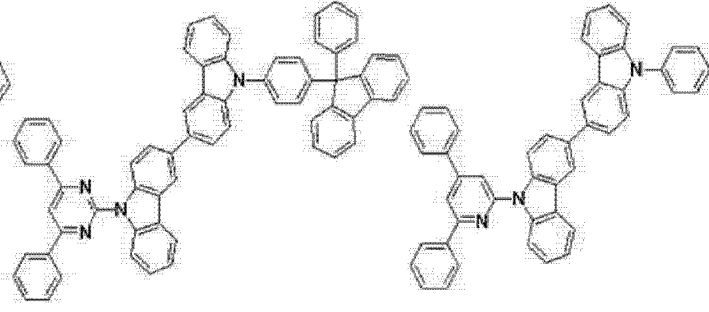
[化学式 A-37]
