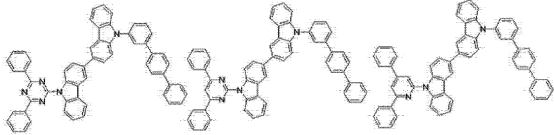
[化学式 A-22]
