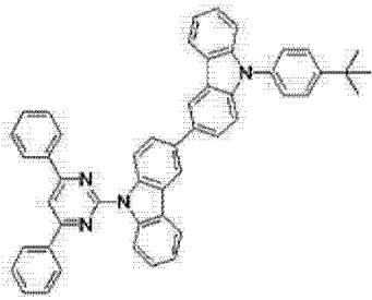
[化学式 B-15]
