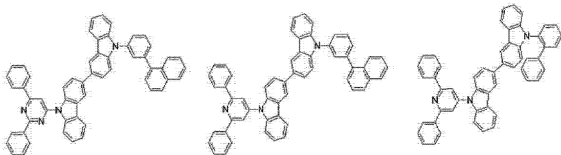
[化学式 A-31]
