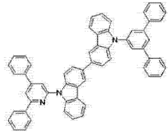
[化学式 A-15]
