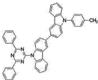
[化学式 B-4]
