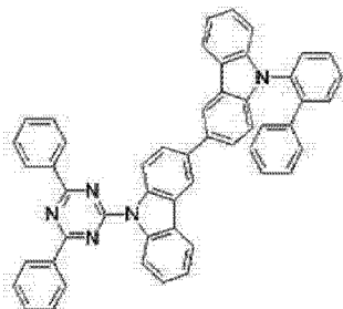
[化学式 A-19]
