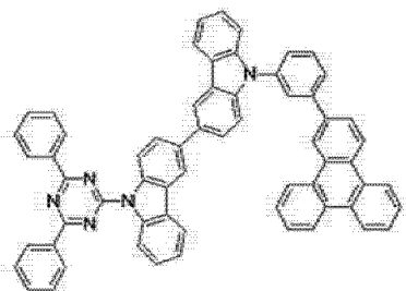
[化学式 A-34]
