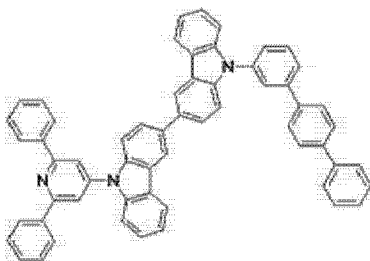
[化学式 A-26]
