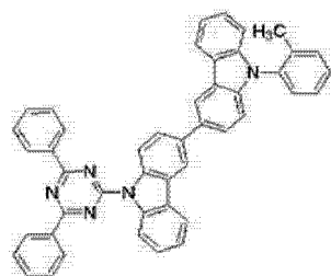
[化学式 B-17]
