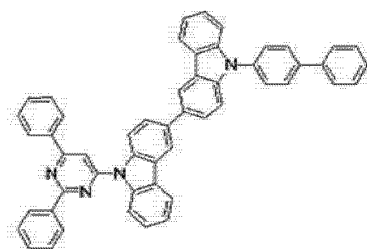
[化学式 A-7]
