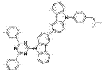
[化学式 B-23]
