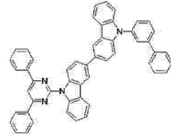
[化学式 A-11]
