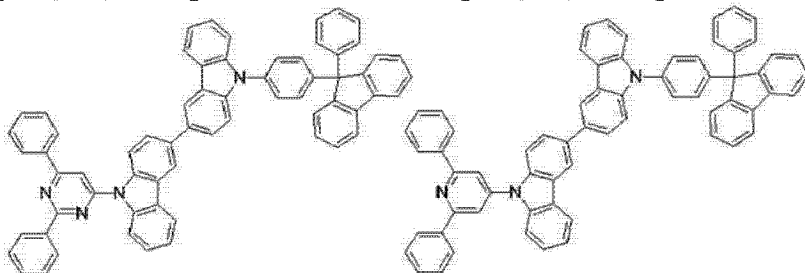
[化学式 A-38]
