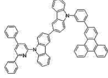
[化学式 A-33]
