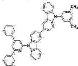
[化学式 B-8]
