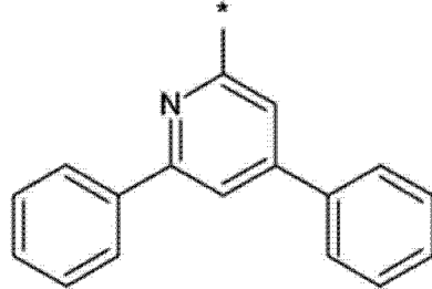
[化学式 6]
