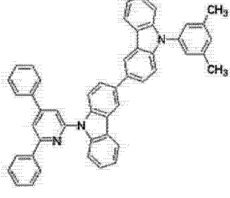
[化学式 B-8]
