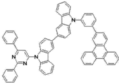
[化学式 A-36]
