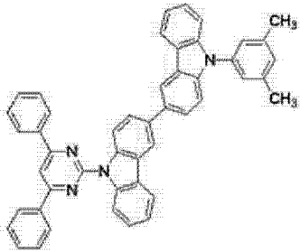
[化学式 B-10]
