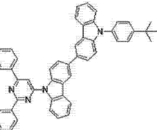
[化学式 B-22]
