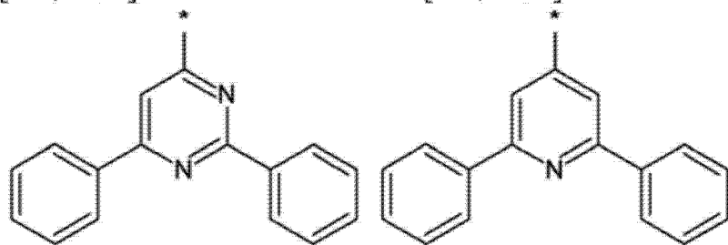
[化学式 6]
