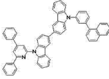
[化学式 A-30]
