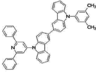
[化学式 B-12]
