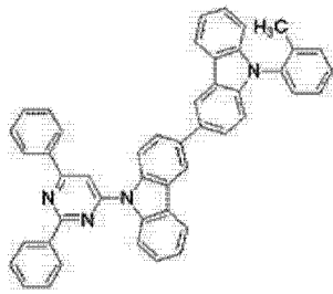
[化学式 B-20]
