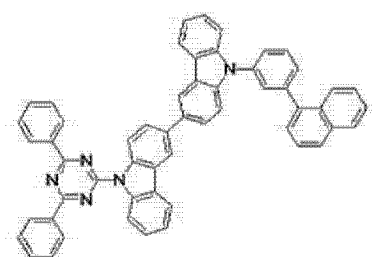
[化学式 A-28]
