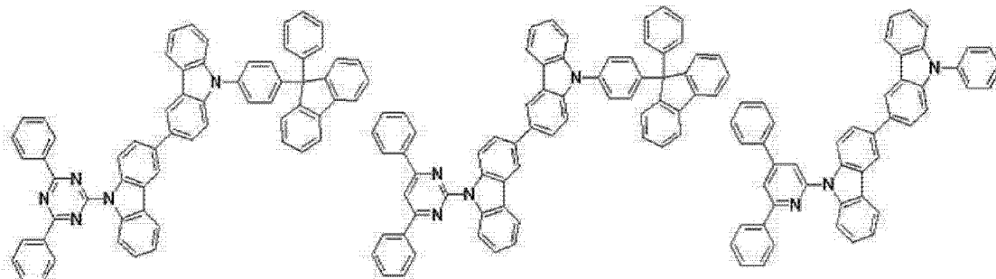
[化学式 A-38]
