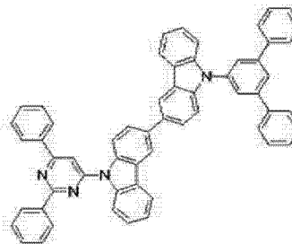
[化学式 A-16]
