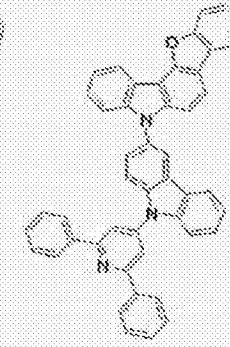
[化学式 B-10]
