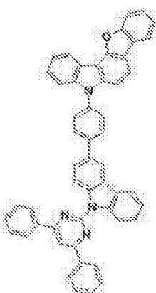
[化学式 B-11]
