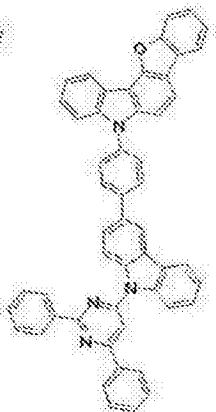
[化学式 B-13]
