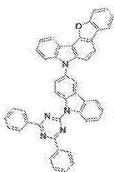
[化学式 B-6]
