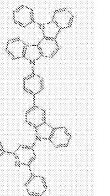
[化学式 C-13]
