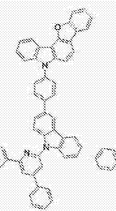
[化学式 B-12]
