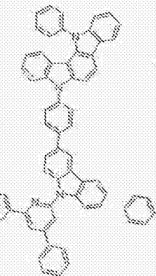
[化学式 C-12]
