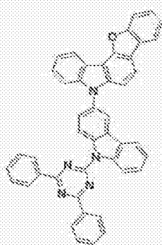
[化学式 B-6]
