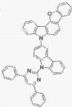
[化学式 B-7]
