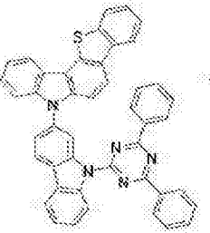
[化学式 A-14]
