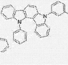
[化学式 C-15]
