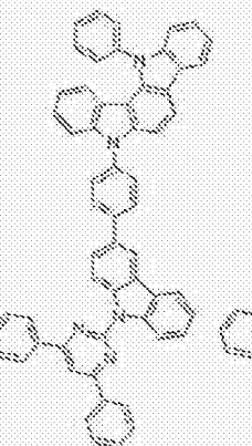
[化学式 C-7]
