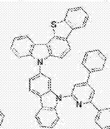
[化学式 A-16]
