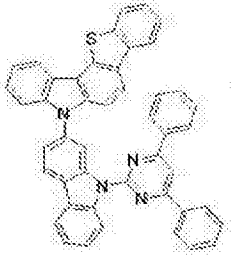
[化学式 A-15]
