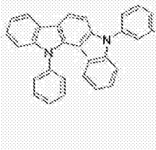
[化学式 C-14]
