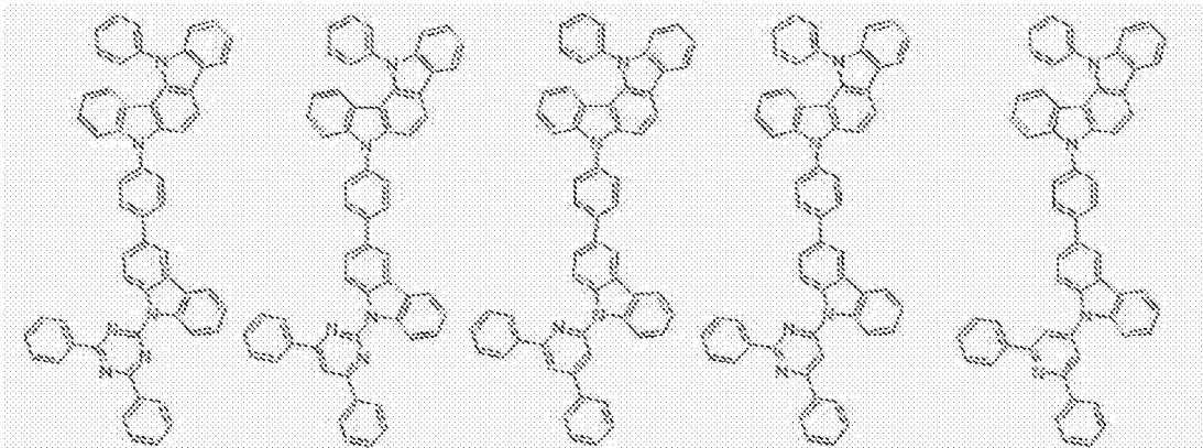
[化学式 C-11]
