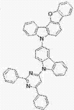
[化学式 B-9]
