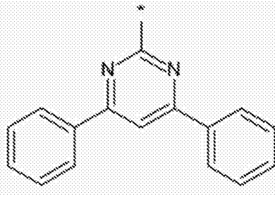
[化学式 9]
