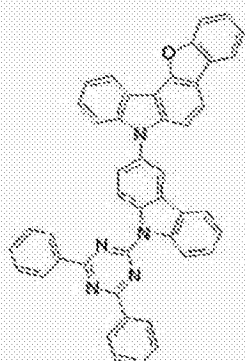
[化学式 B-6]
