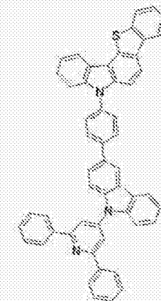
[化学式 A-13]
