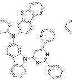
[化学式 A-17]
