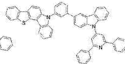
[化学式 A-17]
