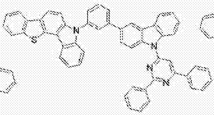
[化学式 A-16]
