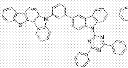
[化学式 A-14]
