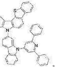
[化学式 A-18]
