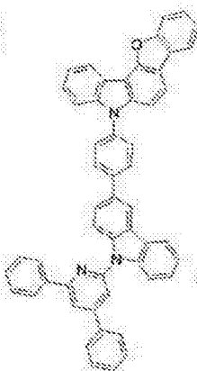
[化学式 B-12]
