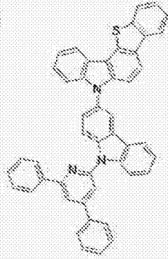
[化学式 A-8]
