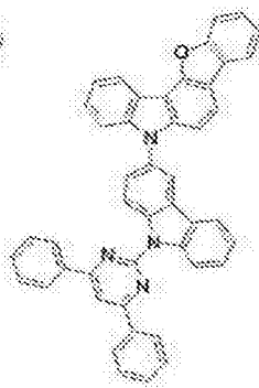
[化学式 B-7]
