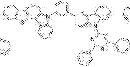
[化学式 A-16]
