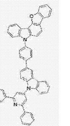
[化学式 B-10]
