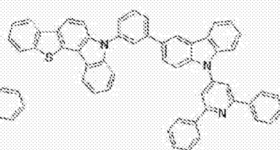
[化学式 A-17]
