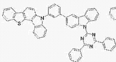
[化学式 A-14]
