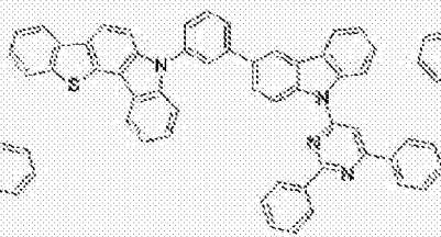
[化学式 A-15]
