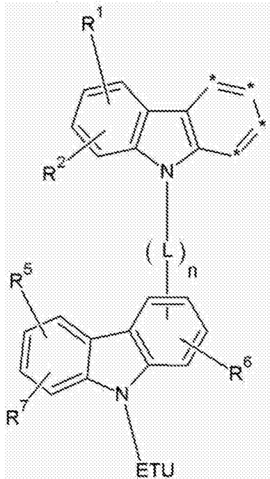
[化学式 1]
