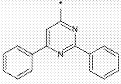
[化学式 10]
