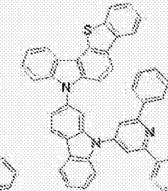
[化学式 A-18]
