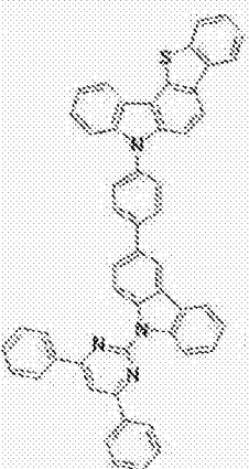
[化学式 A-11]
