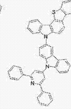
[化学式 A-10]
