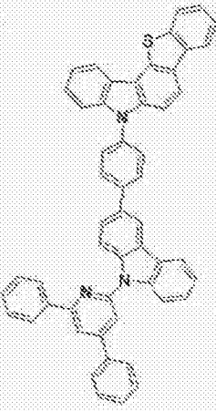
[化学式 A-12]
