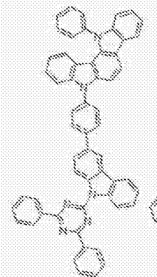
[化学式 C-11]
