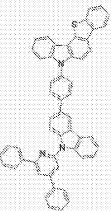
[化学式 A-12]
