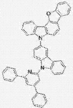
[化学式 B-8]
