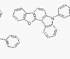
[化学式 B-17]
