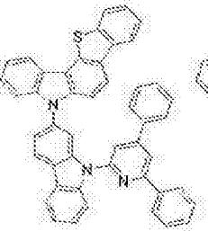
[化学式 A-16]
