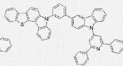
[化学式 A-17]
