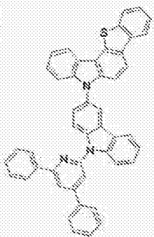
[化学式 A-8]
