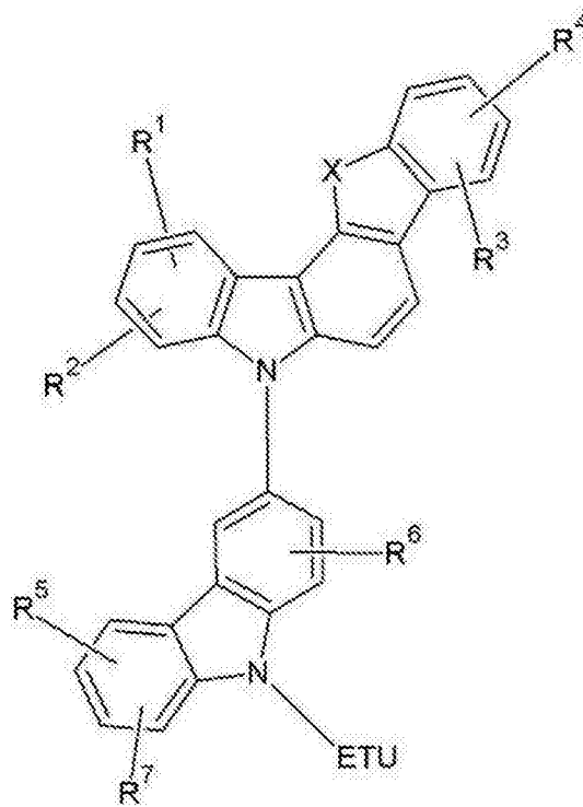
[化学式 5]
