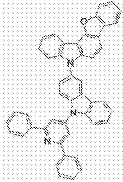
[化学式 B-10]
