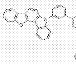
[化学式 B-14]
