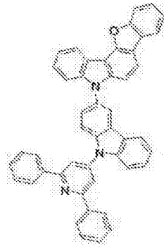
[化学式 B-10]
