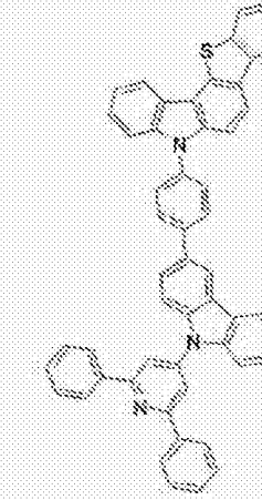
[化学式 A-13]
