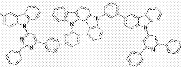
[化学式 C-16]
