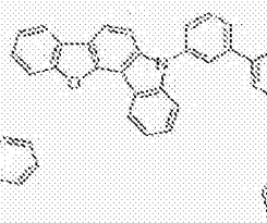
[化学式 B-15]
