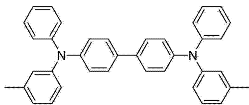
TPD
