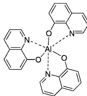
Alq3
