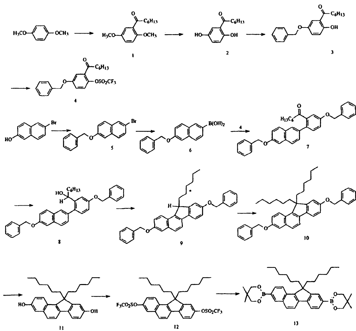
反应方案 1
