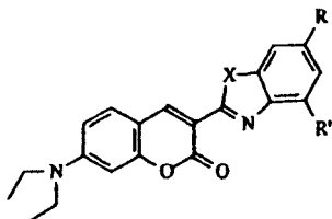
FD 13 R = R' = H, X = O
