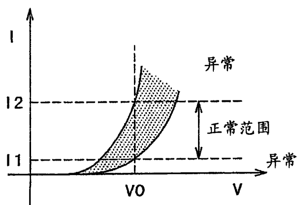
恒定电压驱动检测时的正常范围
