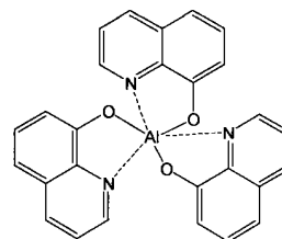
Alq3
