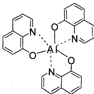
Alq3
