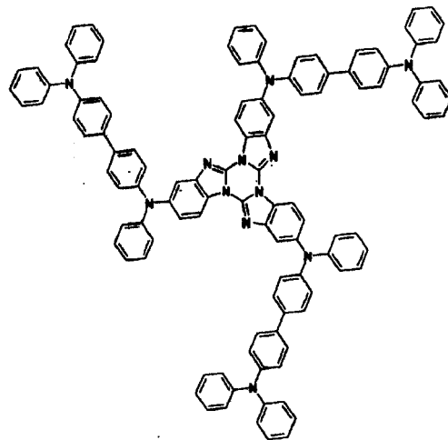
[通式1-42]
