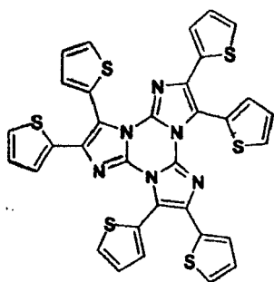
[通式1-19]
