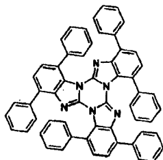
[通式 1-36]
