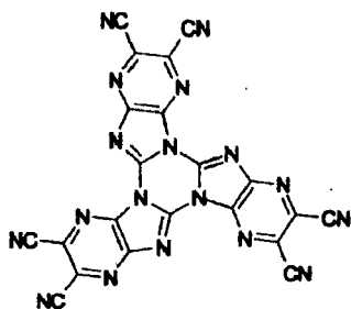
[通式 1-13]
