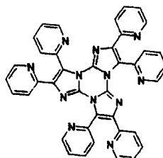
[通式 1-9]
