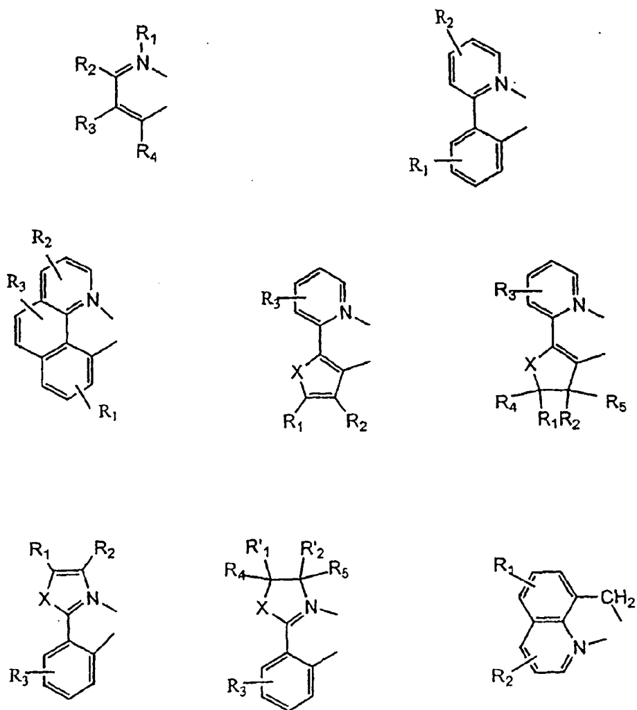
普通单阴离子双齿碳配位配体 I
