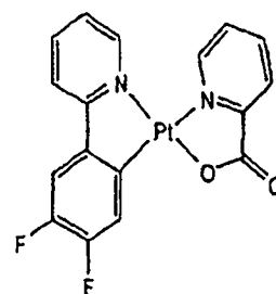
(4,5-F 2 ppy)Pt(pico)
