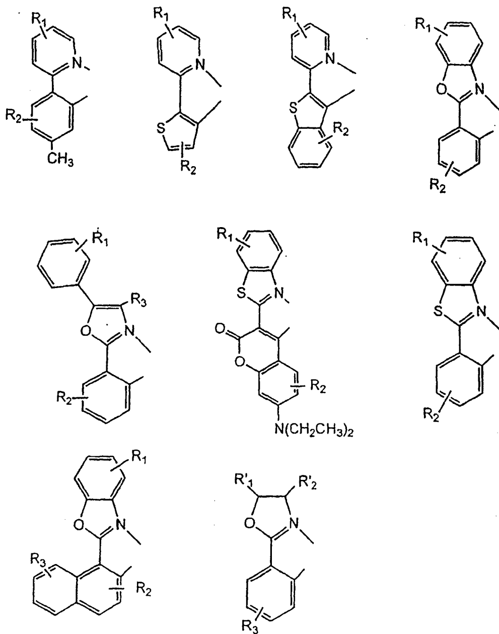
普通单阴离子双齿碳配位配体II
