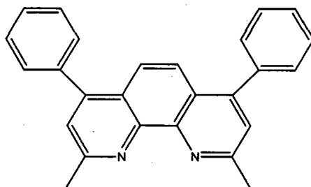
BCP
