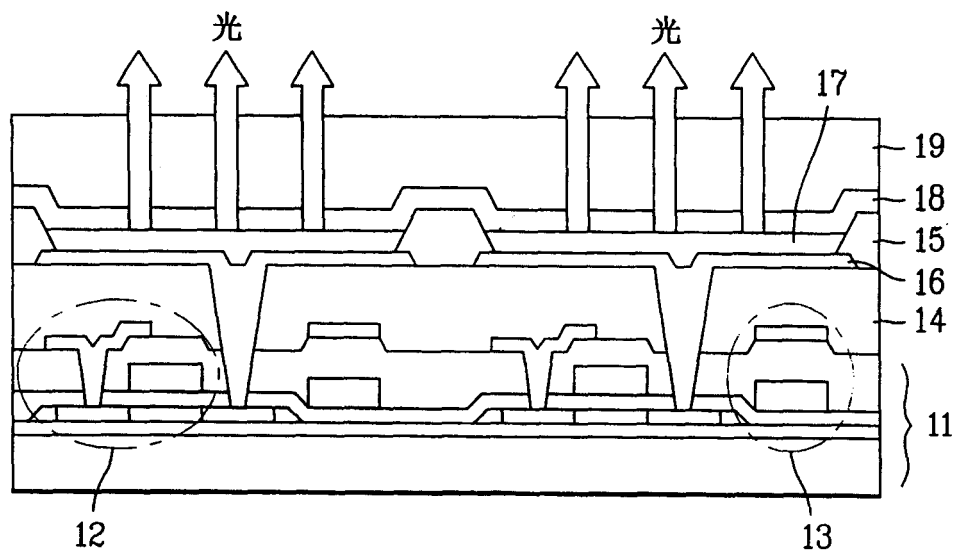
图1 现有技术
