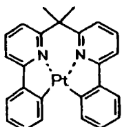
化合物 (79)
