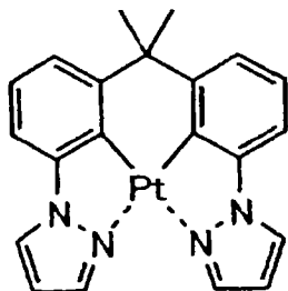
化合物 (227)
