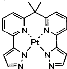
化合物 (218)
