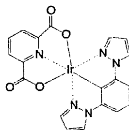
化合物 (160)
