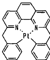
化合物 (47)
