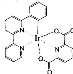
化合物 (115)
