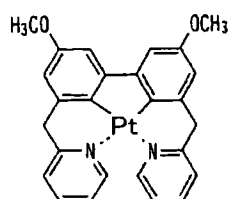
化合物 (37)
