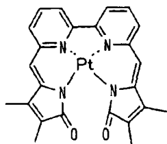
化合物 (24)
