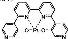
化合物 (205)
