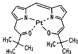
化合物 (28)
