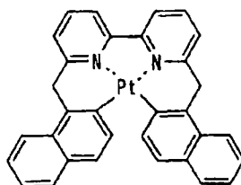
化合物 (46)
