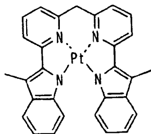
化合物 (62)
