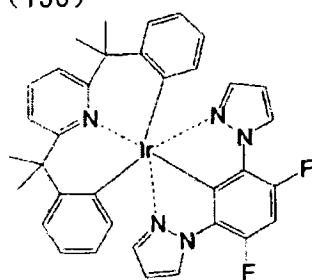
化合物 (156)
