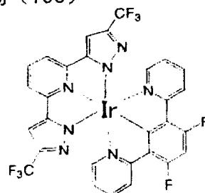
化合物 (107)
