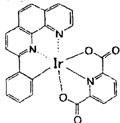
化合物 (121)
