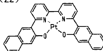
化合物 (22)
