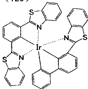
化合物 (130)
