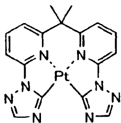
化合物 (215)
