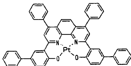
化合物 (16)
