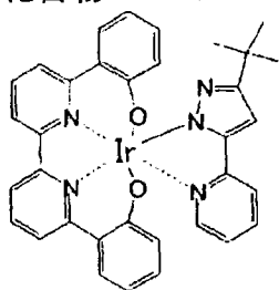
化合物 (119)
