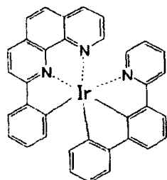
化合物 (121)
