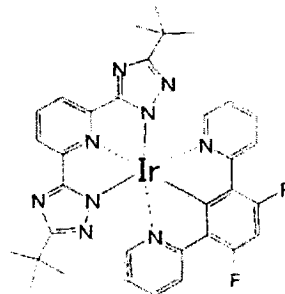
化合物 (107)
