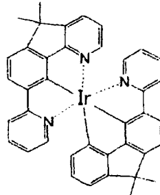
化合物 (125)
