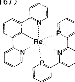
化合物 (168)
