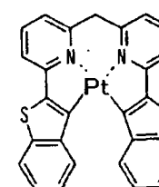
化合物 (52)
