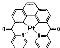
化合物 (35)
