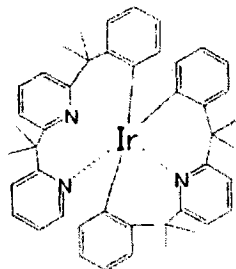
化合物 (102)
