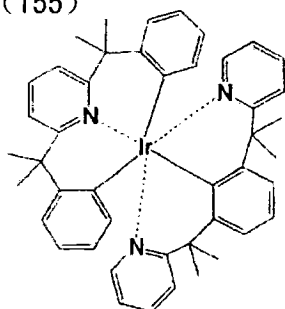
化合物 (155)
