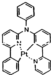
化合物 (140)
