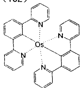
化合物 (132)
