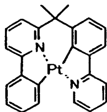
化合物 (139)
