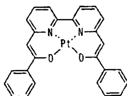
化合物 (151)
