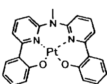
化合物 (70)
