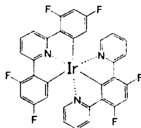
化合物 (104)
