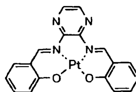
化合物 (93)
