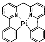
化合物 (50)
