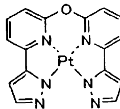
化合物 (223)
