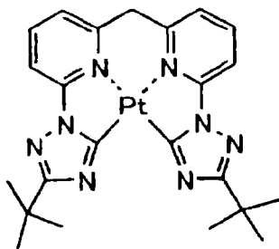
化合物 (219)
