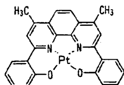
化合物 (14)
