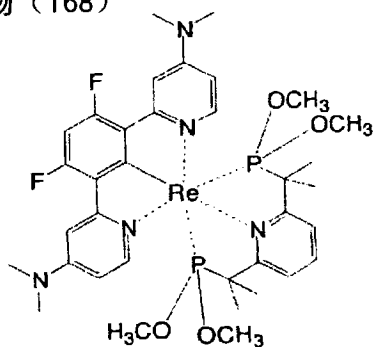
化合物 (168)
