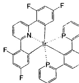
化合物 (175)
