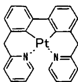
化合物 (34)
