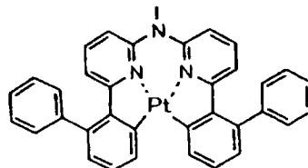
化合物 (86)
