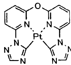
化合物 (217)
