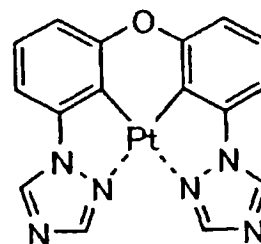
化合物 (232)
