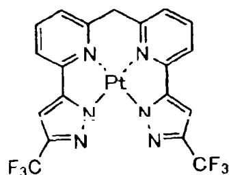
化合物 (222)
