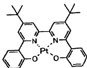
化合物 (65)
