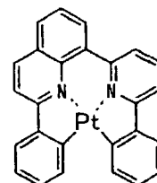
化合物 (57)
