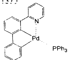
化合物 (137)
