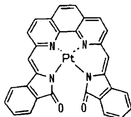
化合物 (25)
