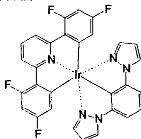
化合物 (172)
