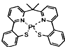
化合物 (69)
