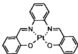
化合物 (88)
