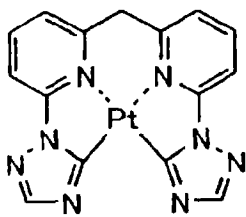
化合物 (216)
