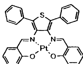
化合物 (91)
