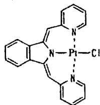
化合物 (146)
