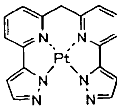
化合物 (222)
