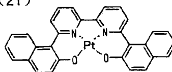
化合物 (21)
