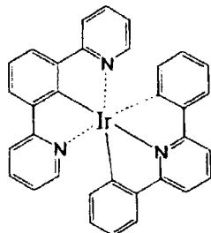
化合物 (110)
