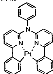
化合物 (82)
