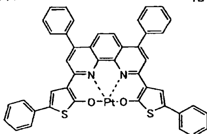
化合物 (205)
