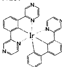
化合物 (125)
