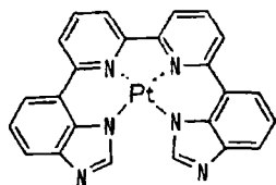
化合物 (3)
