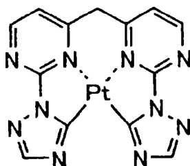
化合物 (228)
