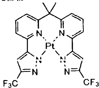
化合物 (221)
