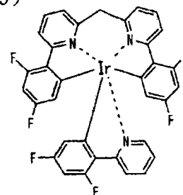
化合物 (152)
