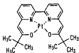
化合物 (150)
