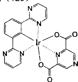
化合物 (129)
