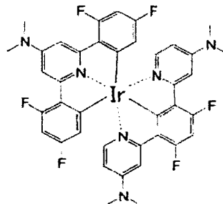
化合物 (105)
