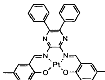
化合物 (94)
