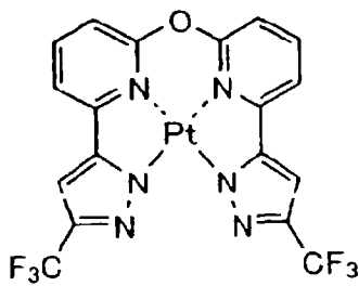
化合物 (223)
