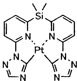
化合物 (235)
