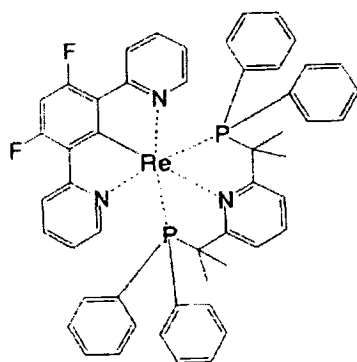
化合物 (165)
