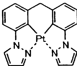
化合物 (231)
