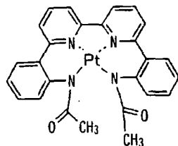
化合物 (5)
