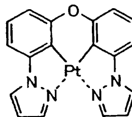
化合物 (232)
