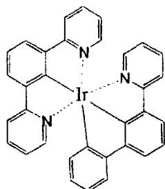
化合物 (109)
