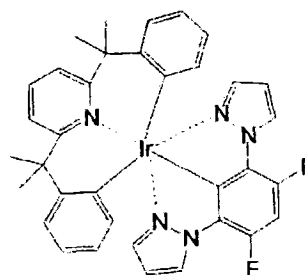
化合物 (166)
