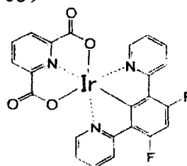
化合物 (106)
