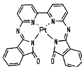
化合物 (26)
