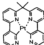
化合物 (84)
