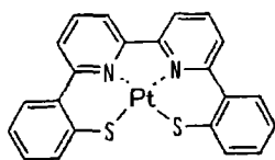
化合物 (2)
