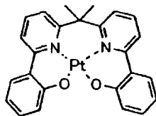
化合物 (66)
