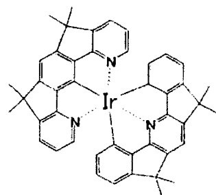
化合物 (100)
