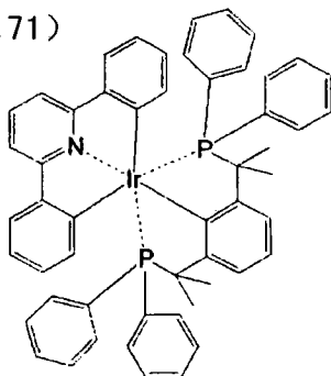
化合物 (175)
