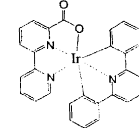
化合物 (117)
