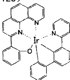
化合物 (124)
