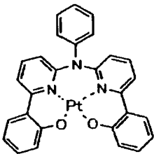
化合物 (70)
