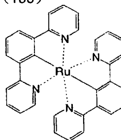
化合物 (134)
