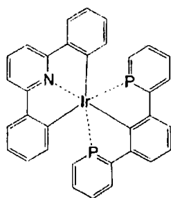
化合物 (170)
