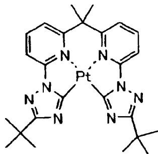
化合物 (218)
