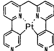
化合物 (51)
