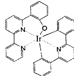
化合物 (116)
