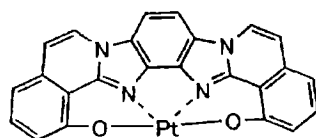
化合物 (183)
