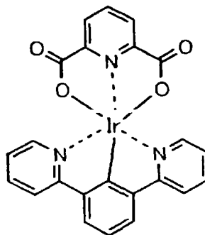
化合物 (143)
