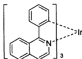
D-4
