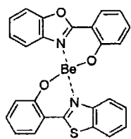
化合物5
