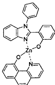
化合物16
