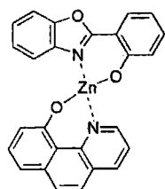
化合物4
