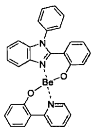
化合物13
