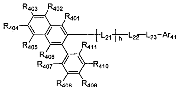
化学式9
