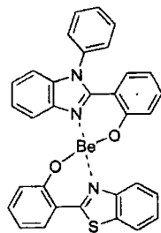
化合物17
