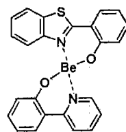
化合物7
