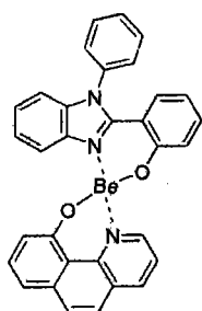
化合物15
