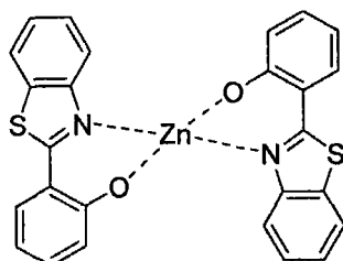
H-26
