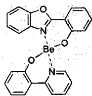
化合物1
