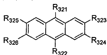
化学式6
