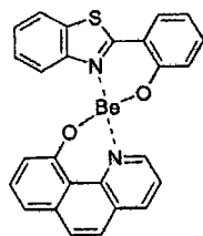
化合物9
