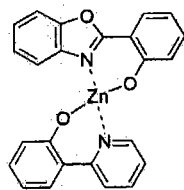
化合物2
