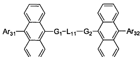
化学式8
