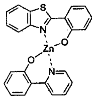
化合物8
