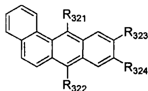
化学式8
