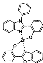
化合物12
