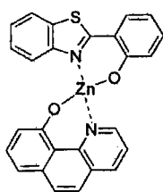
化合物10
