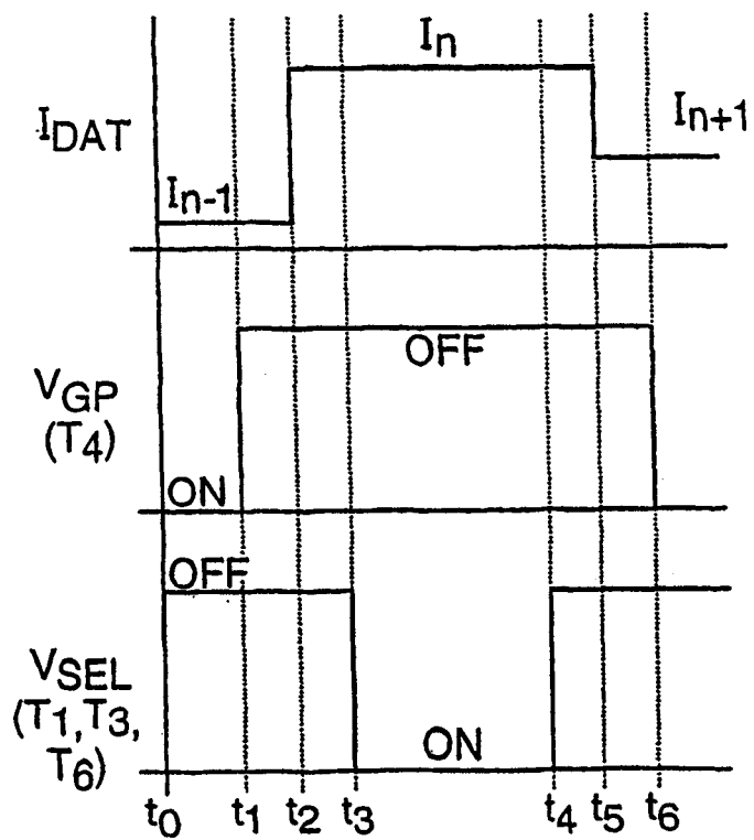
驱动波形
