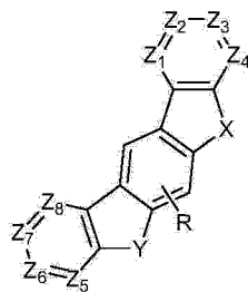
化学式5
