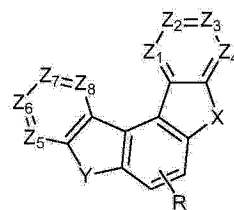
化学式4
