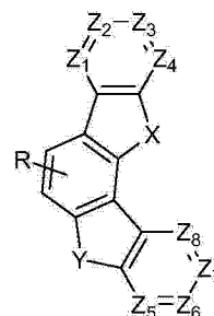
化学式6
