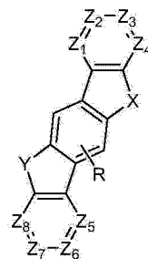
化学式6
