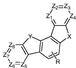
化学式3
