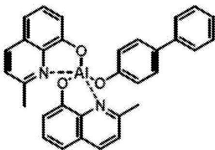
BAlq
