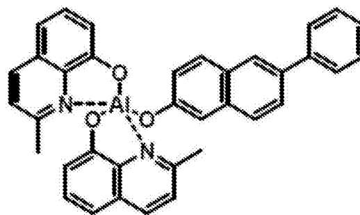
BAlq 衍生物
