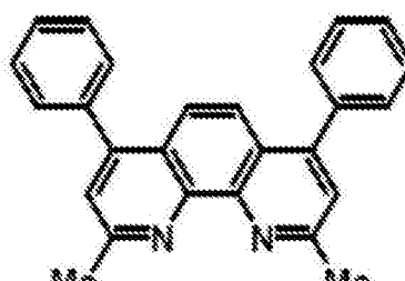
BCP
