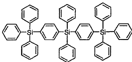
[0296] 比较化合物 3
