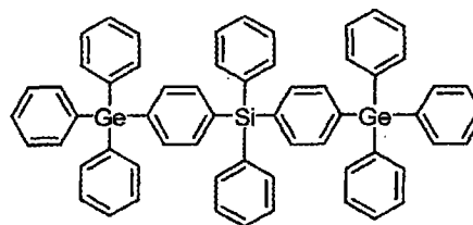
比较化合物 4
