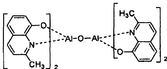
化学式 8
