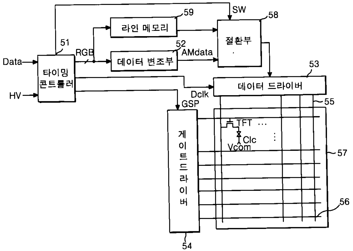
도면5
