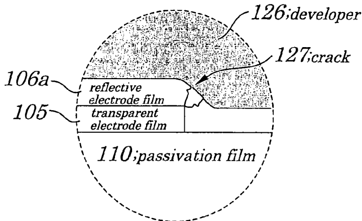
FIG. 31B(PRIOR ART)
