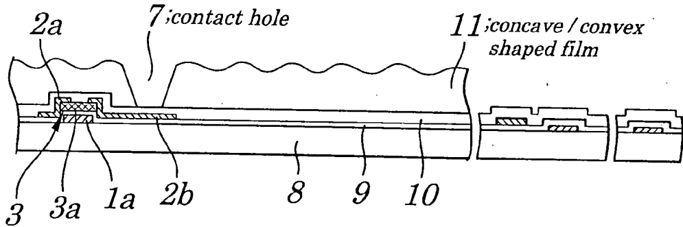
FIG. 14C
