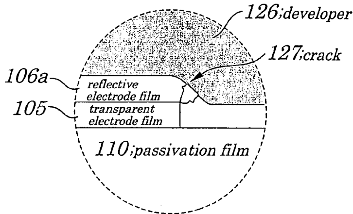
FIG. 31B(PRIOR ART)
