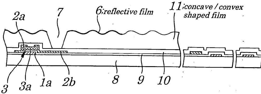
FIG. 3C
