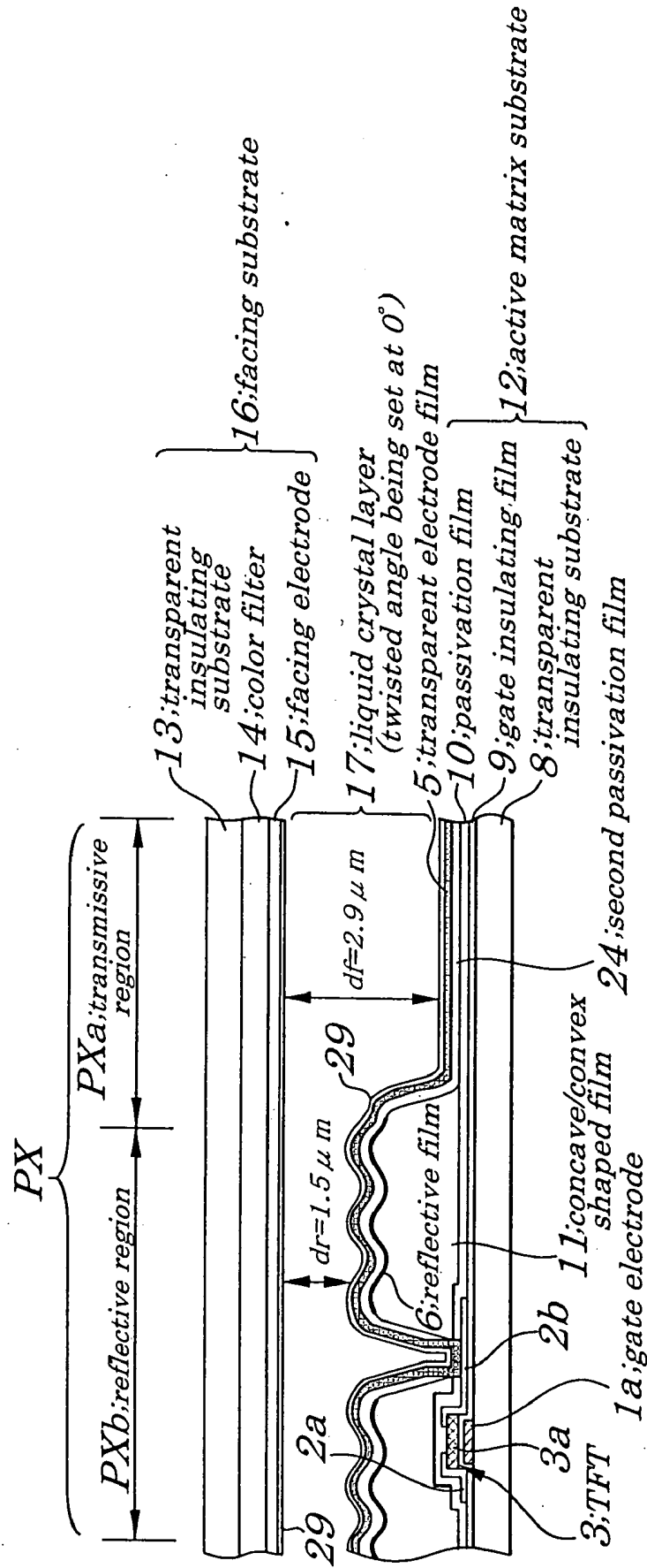
FIG. 6
