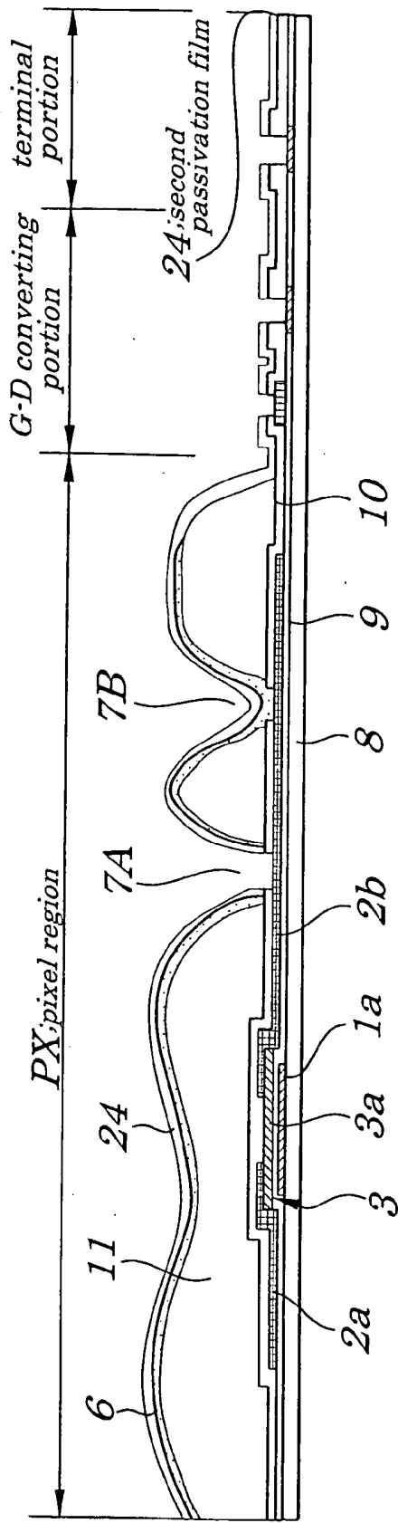
FIG. 29A
