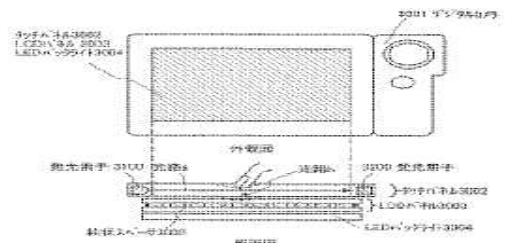
(10) 携帯情報端末装置(タッチパネル式)の外部面および断面図
