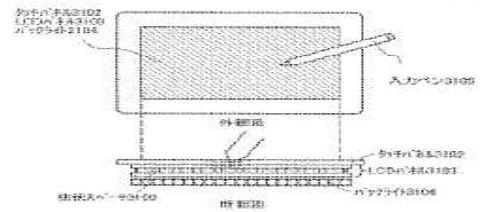
(11) 携帯情報端末装置(ペン入力式タッチパネル)の外部面および断面図
