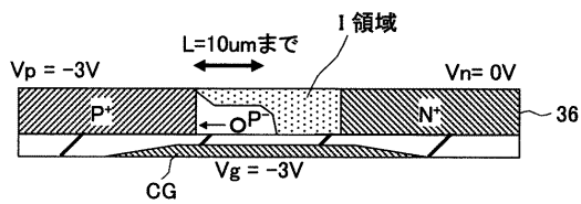
(A) PIN構造
