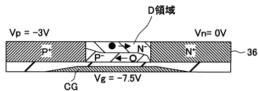
(B) PDN構造
