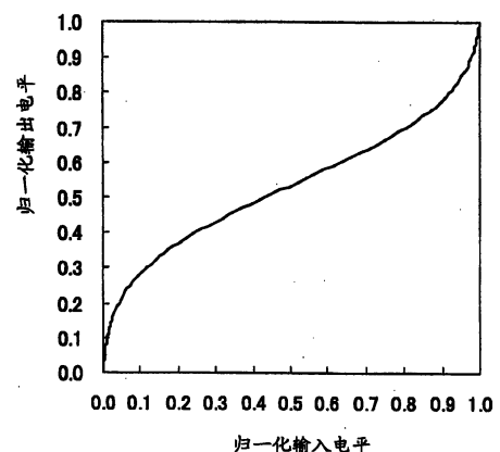
S形反函数
